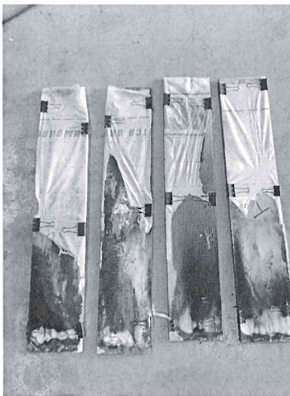
Фото. Образец после испытания на горючесть.
